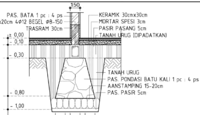
FONDASI SKALA 1 : 30
